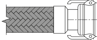
52909-C Raccord à came coupleur
